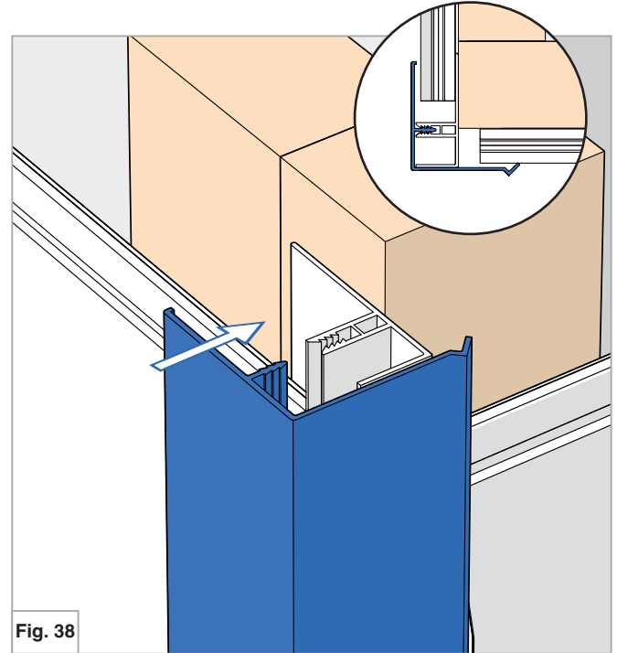
Fig. 38 Angle extérieur BRA3
