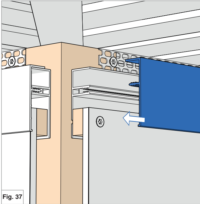
Fig. 37 Finition haute BRF3
