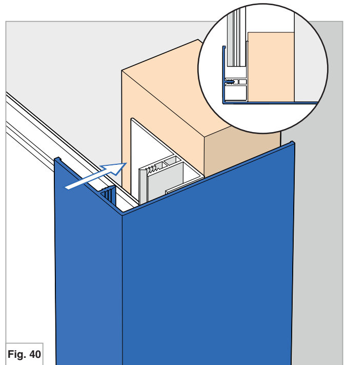
Fig. 40 Finition d'arrêt de bardage BRC3/BRL3
