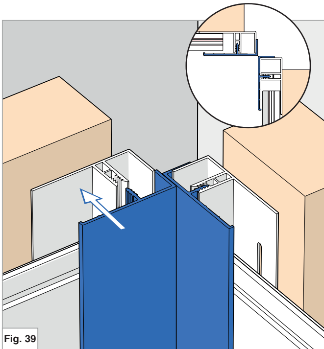
Fig. 39 Finition intérieure BRF3
